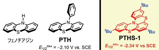
図1 フェノチアジン有機フォトレドックス触媒の分子構造
